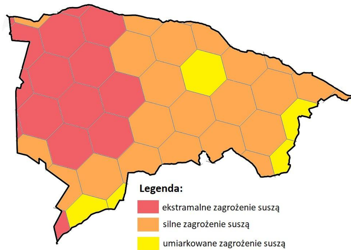
Mapa 5 Mapa łącznego zagrożenia suszą suma klas zagrożenia suszą rolniczą, hydrologiczną i hydrogeologiczną – ocena w siatce pól podstawowych
