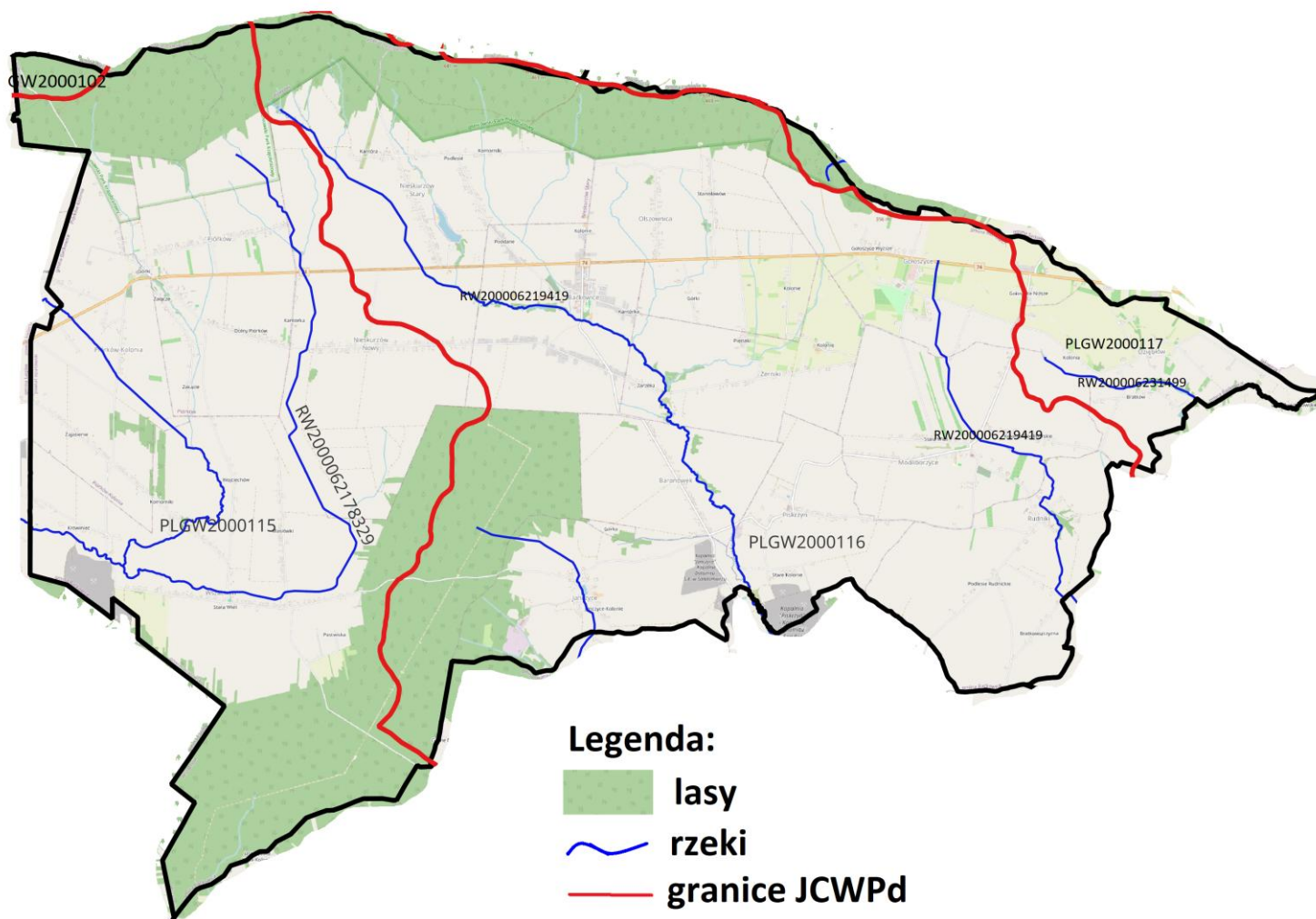
Mapa 4 Położenie gminy Baćkowice na tle obszarów JCWP i JCWPd
