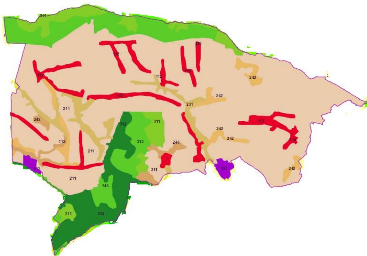
Mapa 2 Pokrycie terenu w gminie Baćkowice
